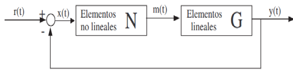
Figura 2: Sistema no lineal con parte lineal
