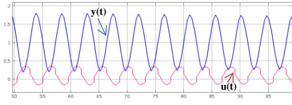
Figura 5: Ciclo límite sinusoidal obtenido con planta \frac{10 e^{-0.7s}}{(0.4s+1)(2s+1)} y PI+CI con p_r = 0.6, \tau_i = 1, k_c = 0.2 .
